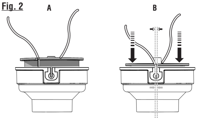
A - Insert line into string head (insérer dans l'extrémité de la chaîne, insérez en el cabezal del hilo) B - Push down and twist to align (pousser vers le bas et tordre pour aligner, empujar hacia abajo y girar para alinear)
